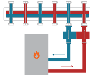
Горизонтальный монтаж гидравлического разделителя
