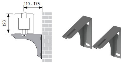
EWG25.001, крепеж распределительного коллектора серий СМАРТБОКС 3.5/6.5
